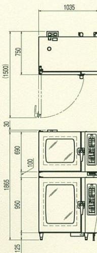
SCOS-6610RH-R(L) 1/1ホテルパン 6段×2
