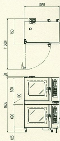
SCOS-6610RH-R(L) 1/1ホテルパン 6段×2
