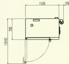
SCOS-2010RH-R(L) 1/1ホテルパン 20段
