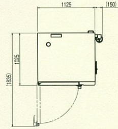
SCOS-1220RH-R(L) 2/1ホテルパン 12段
