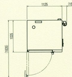
SCOS-2020RH-R(L) 2/1ホテルパン 20段
