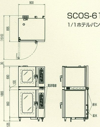
SCOS-6611RH-R(L) 1/1ホテルパン 6段×2
