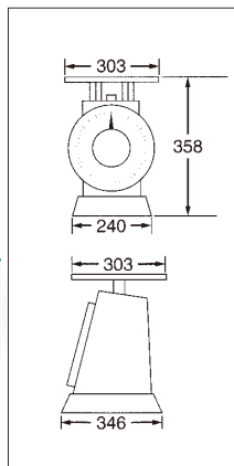
● 寸法図 (単位mm)
